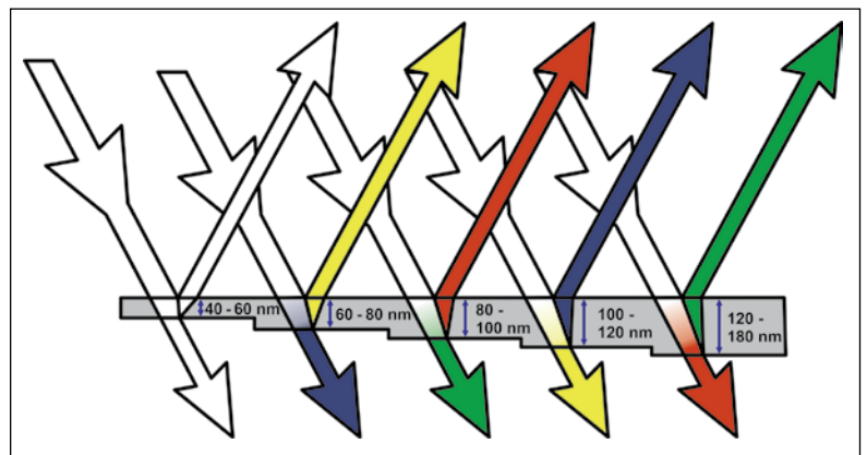
Bild 3: Die Schichtdicke der Metalloxydbeschichtung und der kombinierte Einstrahlungs- und Betrachtungswinkel bestimmen die optische Weglänge und somit die sich ergebenden Interferenzfarben in Reflexion und Transmission
