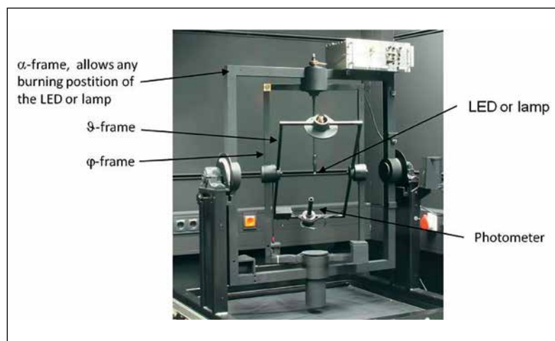
Bild 6: Kleines Kardan-Goniophotometer 1982–2007
