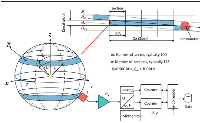
Bild 5: Signalfluss
