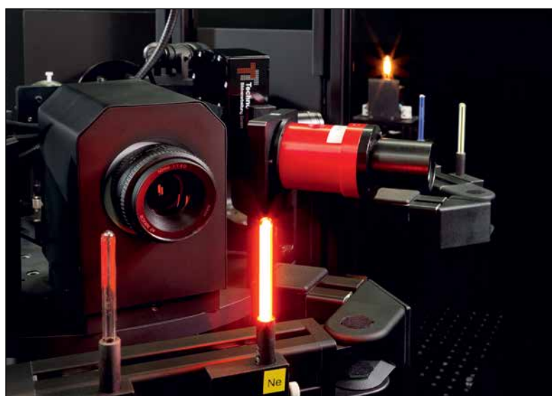
Bild 10: Entladungslampen mit verschiedenen Gasfüllungen dienen der Wellenlängenkalibrierung der Spektrometer. Im Hintergrund ist eine Bestrahlungsstärke-Normlampe für die spektrale Empfindlichkeitskalibrierung zu sehen.
