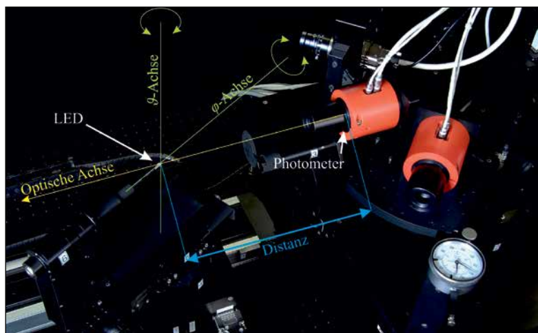
Bild 8: Goniophotometer für photometrische Messungen an Kleinleistungs-LEDs
