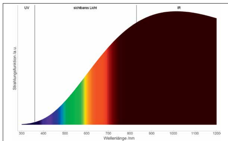
Bild 1: Spektrale Verteilung einer Glühlampe und spektraler Hellempfindlichkeitsgrad ( V(\lambda) -Funktion)
