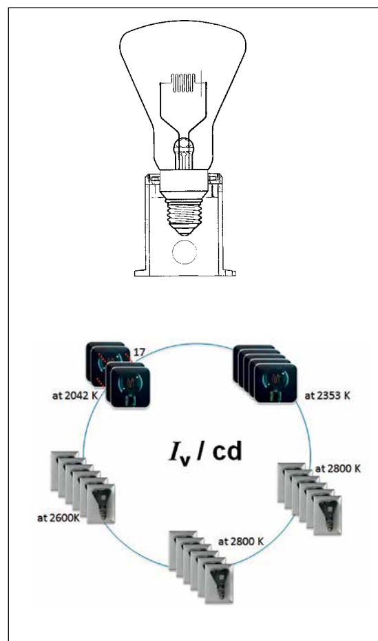
Bild 3: Lichtstärke-Normallampe WI41/G mit PTB-Spezialsockel (oben) sowie verschiedene Lichtstärke-Normallampengruppen zur Bewahrung und Weitergabe der Lichtstärke-Einheit (unten)
