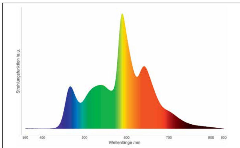
Bild 3: Exemplarische spektrale Verteilung einer weißen OLED
