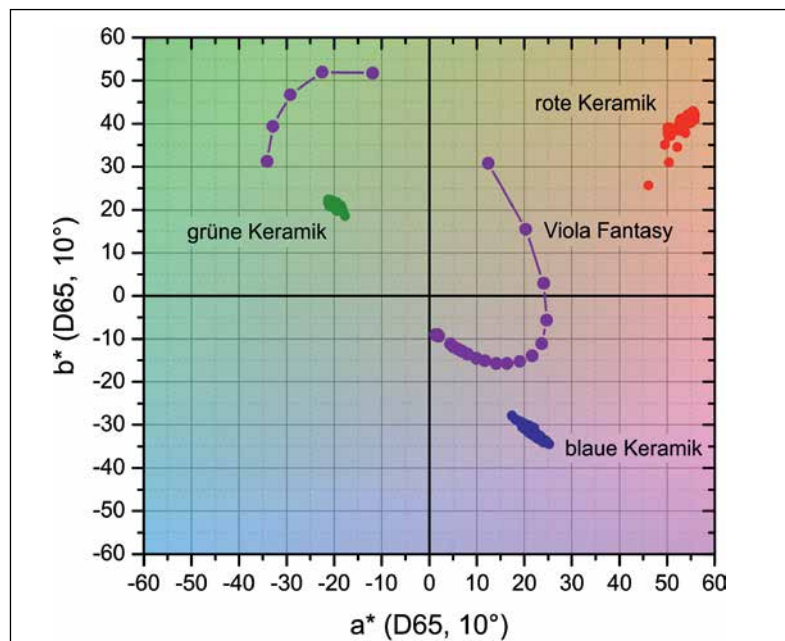
Bild 6: CIELab Farbkordinaten einer winkelabhängigen Reflexionsmessung an vier verschiedenen Proben: drei Keramiken der Farben rot, grün, blau und eine Effektpigmentlackierung mit Merck Colorstream® Viola Fantasy. Das untergelegte Farbschema zeigt näherungsweise die den Koordinaten entsprechende Farbe.
