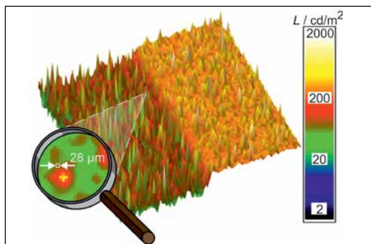
Bild 8: Visualisierung des Sparkling-Effektes von Xirona®-Volcanic-Sparks-Pigmenten als Falschfarbendarstellung der orts aufgelösten Leuchtdichte. Die „Nadeln“ zeigen die Position der Pigmente an.
