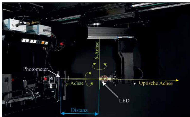
Bild 9: Goniophotometer für photometrische Messungen an Hochleistungs-LEDs
