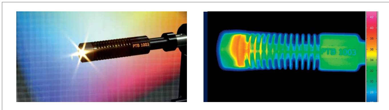
Bild 5: Temperaturgeregeltes LED-Transferrnormal auf Basis von Hochleistungs-LEDs mit Lichtströmen von bis zu 100 Lumen. Im rechten Bild ist die Temperaturverteilung in Grad Celsius während des Betriebs abgebildet.
