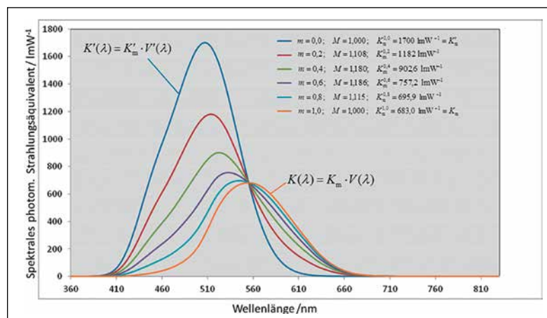
Bild 2: Die mesopische Hellempfindlichkeitsfunktionen V_{\text{mes}}(\lambda) für unterschiedliche Adaptionsniveaus mit deren zugehörigen maximalen Strahlungsäquivalenten
