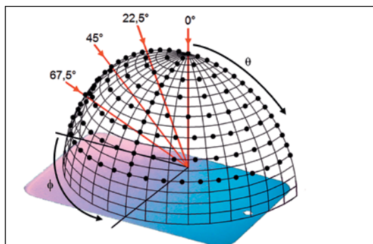
Bild 9: Beispielgeometrien zur Messung der winkelabhängigen Reflexionseigenschaften. Realisiert wurden 4 Einstrahlungsrichtungen (rote Pfeile) mit jeweils 114 Reflexionswinkeln (schwarze Punkte) im Bereich der Viertelkugel oberhalb der Probenoberfläche.
