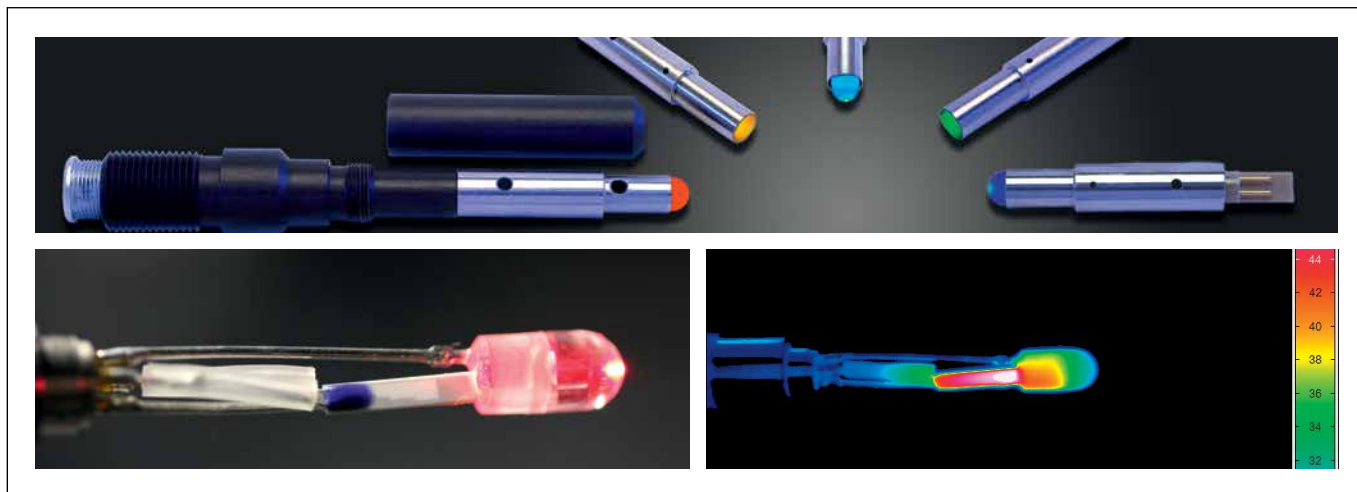
Bild 4: Temperaturgeregeltes LED-Transferrnormal auf Basis von Kleinleistungs-LEDs mit Lichtströmen von bis zu 10 Lumen.
